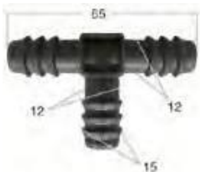
Conexión Tipo "T" Diámetro: 15mm
