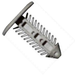
Chilillo Universal Ford h: 23mm Diámetro: 8mm
