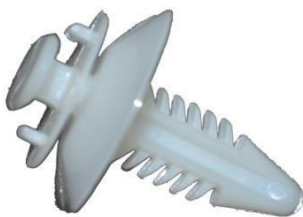
Grapa Para Puertas Chevrolet h: 27mm Diámetro: 8mm
